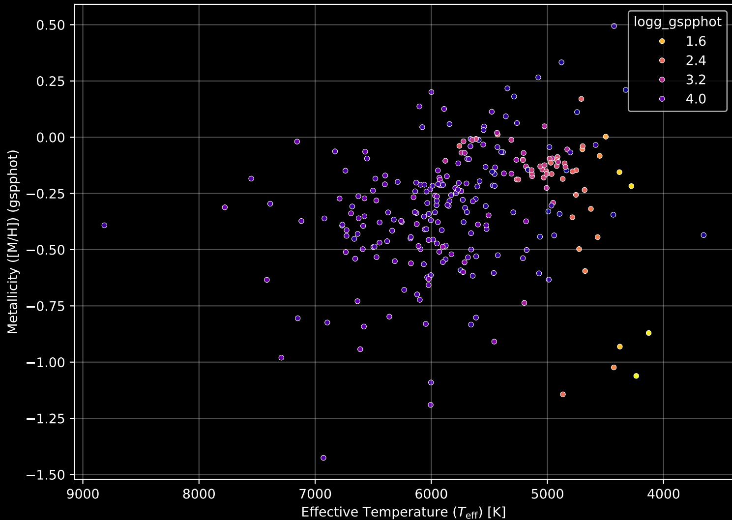
GALAH DR4 Field: [2858] Stellar Population Parameters (n= 267)
