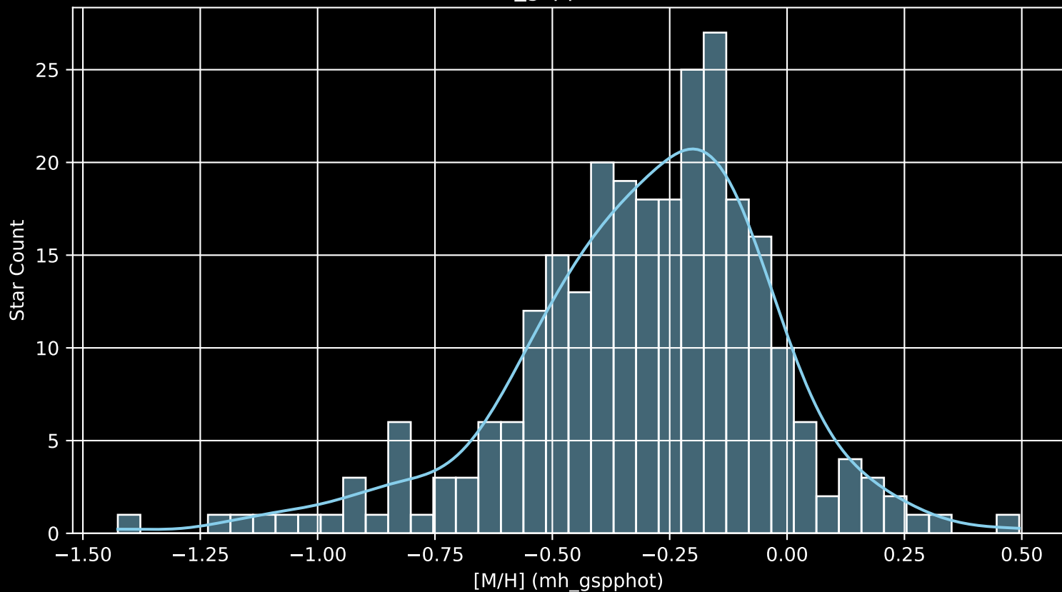
GALAH DR4 Field: [2858] [M/H] (mh_gspphot) (n= 267)
