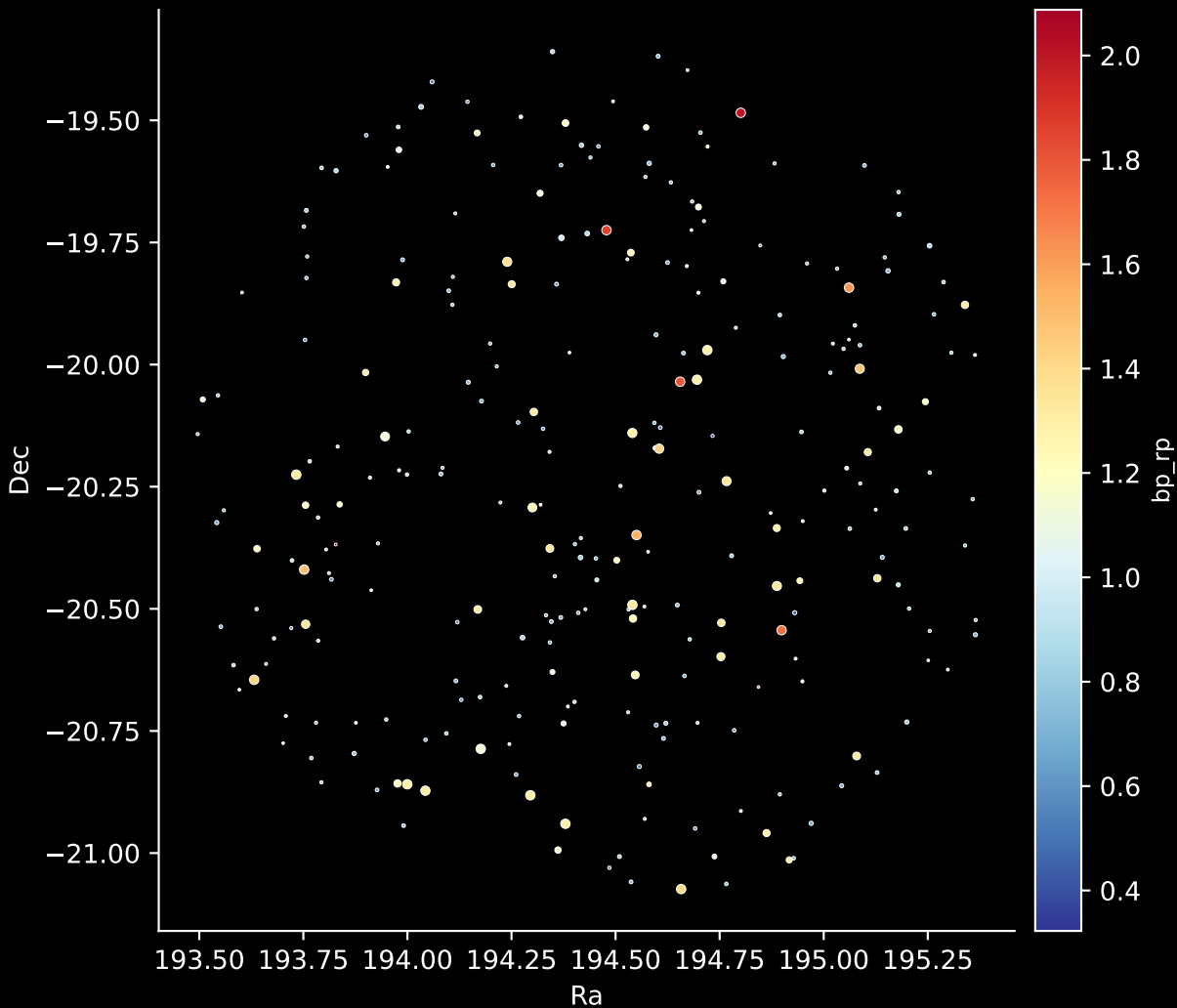
GALAH DR4 Field: [2858] Stars: 267
