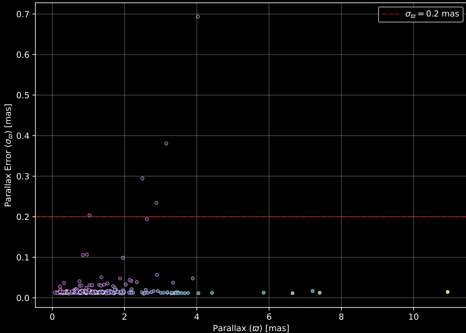
GALAH DR4 Field: [2858] Parallax Quality (n= 267)
